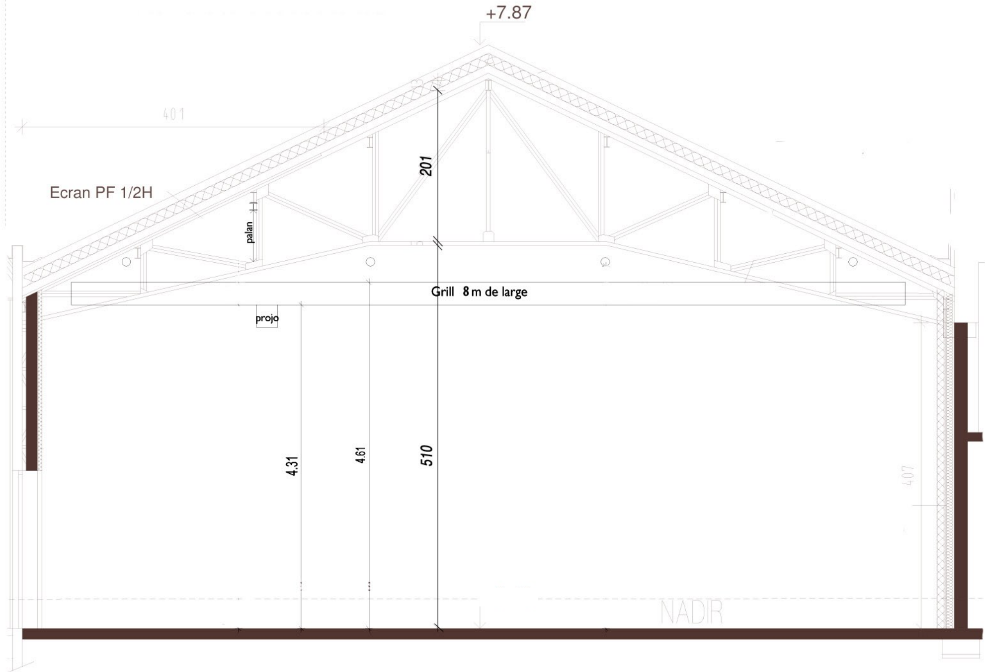
Coupe Nadir - Emprise du grill
